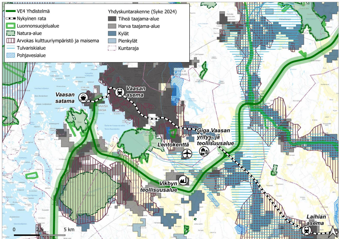
Kuva 28. Linjausvaihtoehto 4 Yhdistelmä.
